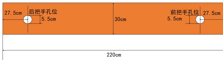
图 1.2: 龙身、龙尾俯视数据图
