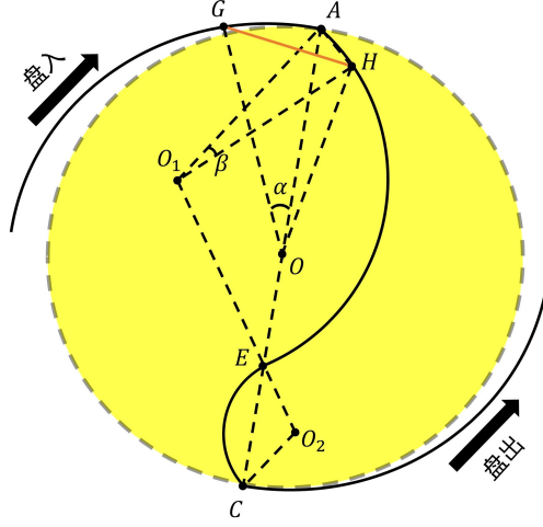
图 4.20: 情况二示意图
