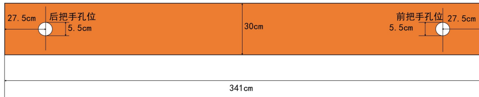
图 1.1: 龙头俯视数据图
